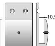
opa 200 w 49 x h 79 x d 22mm w 1,93 x h 3,11 x d 0,87"
