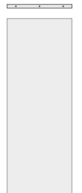
amer 720M w 701 x h 1993 x d 35mm w 27,6 x h 78,47 x d 1,38" w 685 x h 1985 x d 35mm w 26,97 x h 78,17 x d 1,38"
